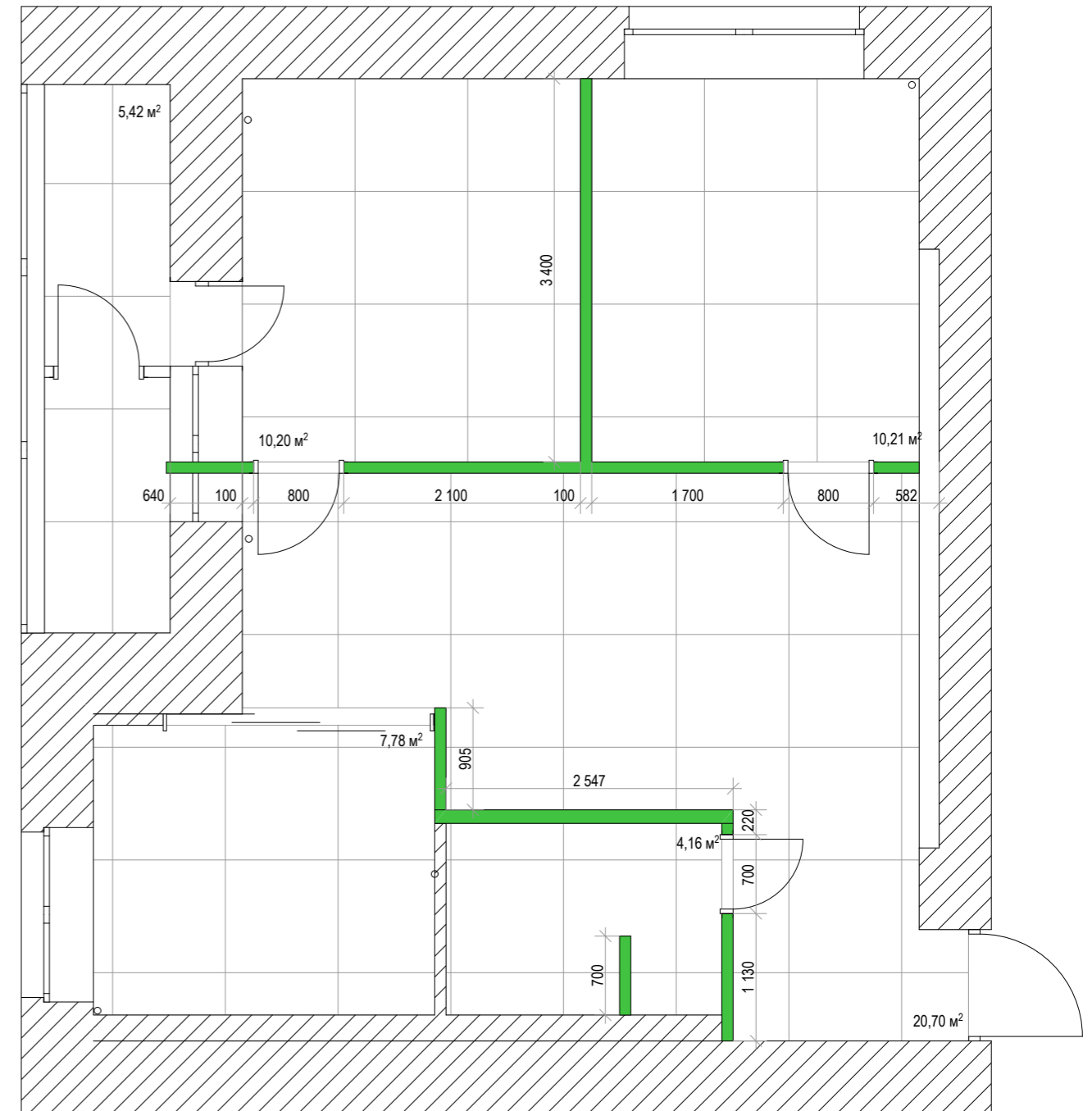
Монтажный план
