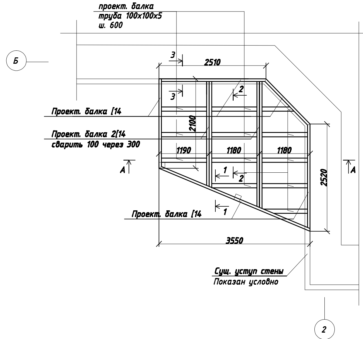
СХЕМА РАСПОЛОЖЕНИЯ МЕТАЛЛИЧЕСКИХ ЭЛЕМЕНТОВ
